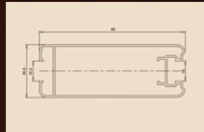
Вертикальный профиль 80*30 - стандартная длина 2700мм, возможно изготовление большей длины под заказ.
